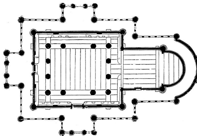
Grunnplanet av stavkirken slik den mest sannsynlig har sett ut; med hevet midt-rom
