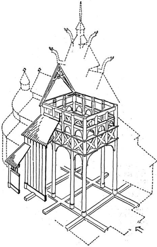
Reisverk konstruksjonen av ny-kirken på Bjerkreim
