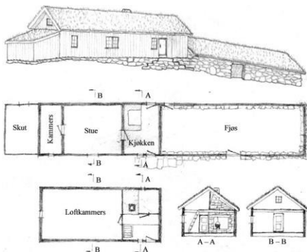
Huset på Østre-tufta, sett fra sør, slik det stod i 1873 da gården ble fraflyttet. Tegning: Paul Tengedal.
